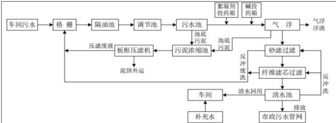
图3-1 污水处理站工艺流程图
