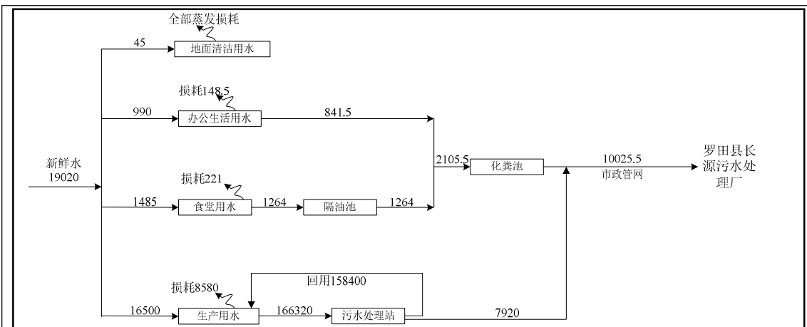
图2-1 水平衡图（一期）（m 3 /a）
