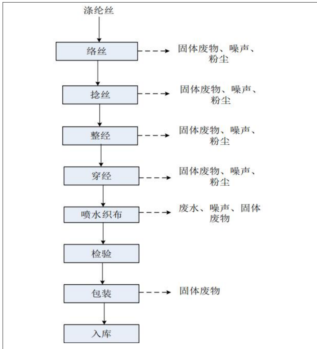
图2-3 化纤布生产工艺流程及产污节点图
